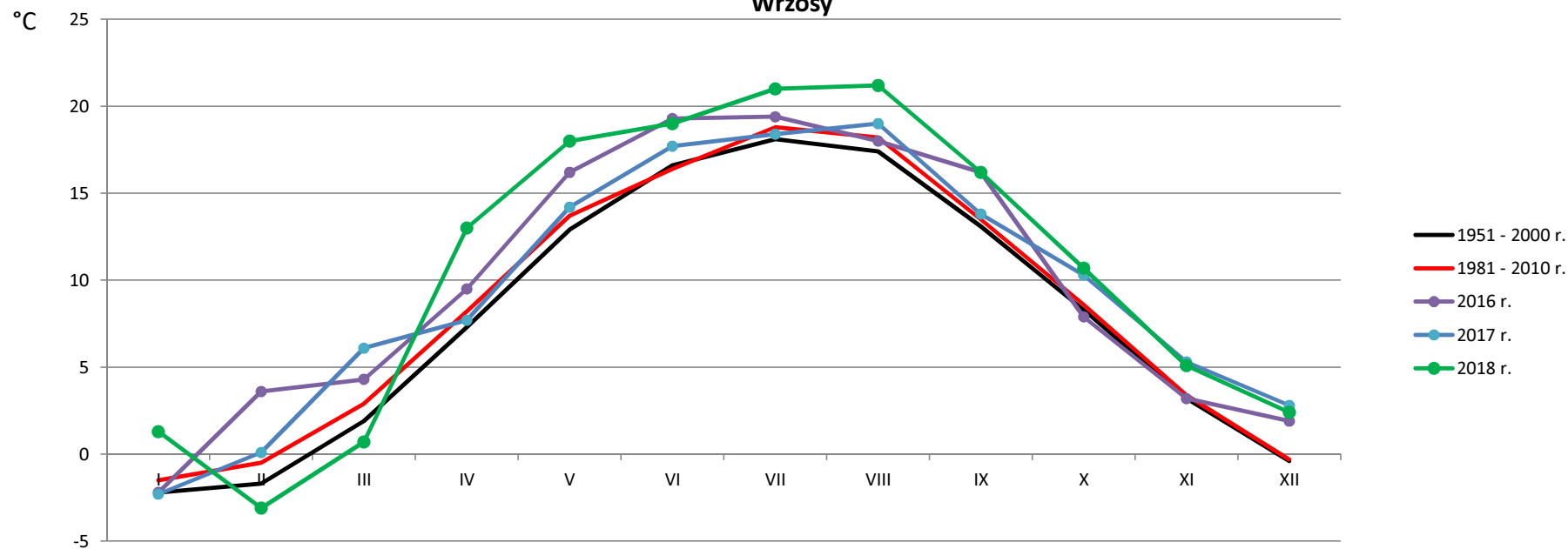
Przebieg roczny temperatury powietrza w Obserwatorium Meteorologicznym Katedry Meteorologii i Klimatologii UMK w 2016, 2017 i 2018 r. na tle wartości wieloletnich (1951-2000 i 1981-2010) ze stacji Toruń-Wrzosy
