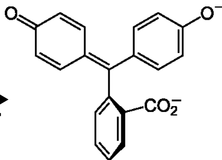
Forma malinowa
