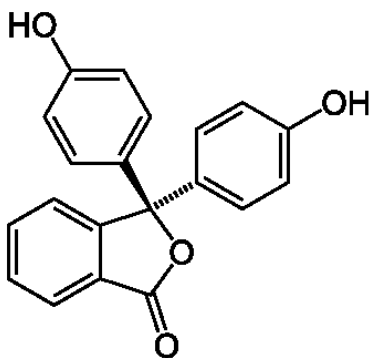
Forma bezbarwna
