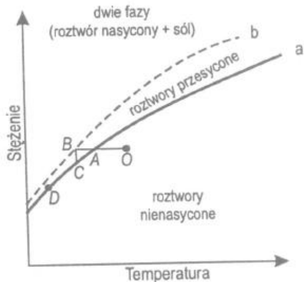
Rozpuszczalność + krystalizacja
