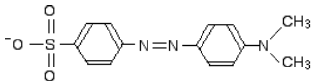
Forma żółta
