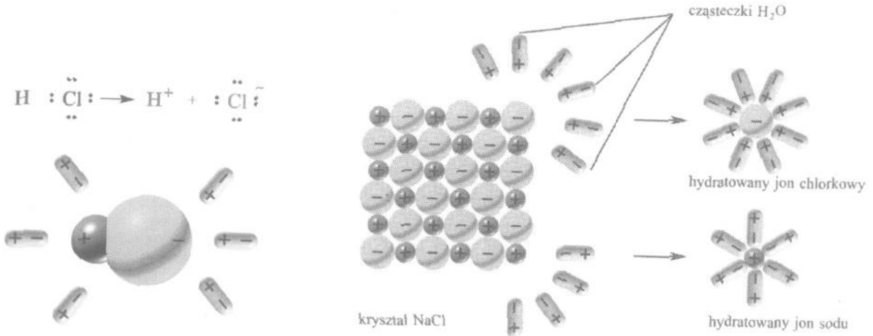
związki kowalencyjne
