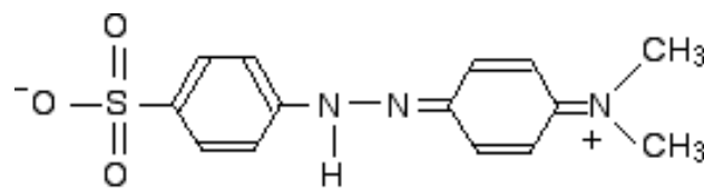
Forma czerwona
